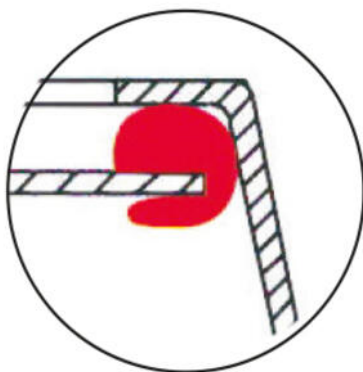
Paknings detalje
