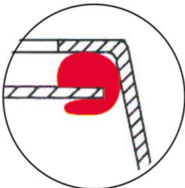
Paknings detalje
